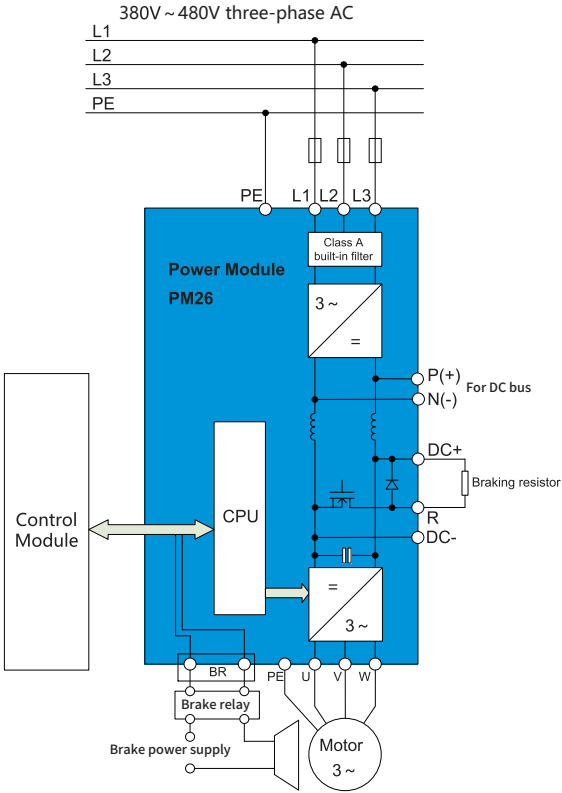
14.3 功率模块电气连接
