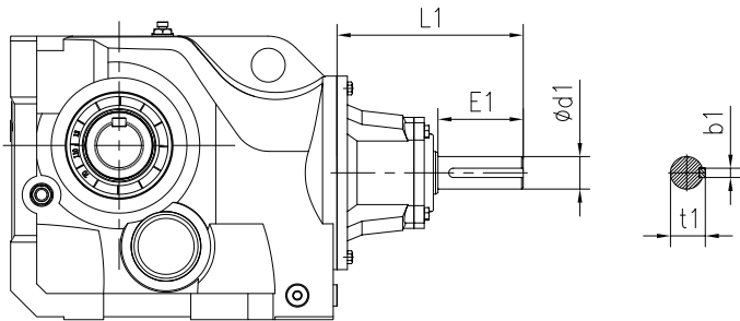
6.4 K系列AE输入轴外形尺寸(mm)
