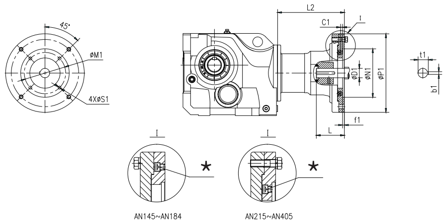
6.3 K系列AN连接 法兰尺寸(mm)
