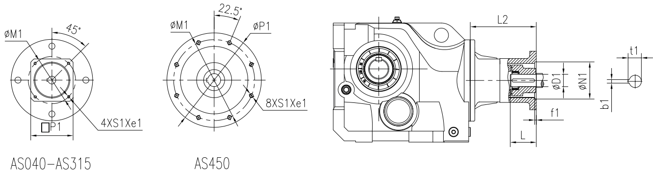
6.2 K系列AS输入 法兰外形尺寸图表(mm)
