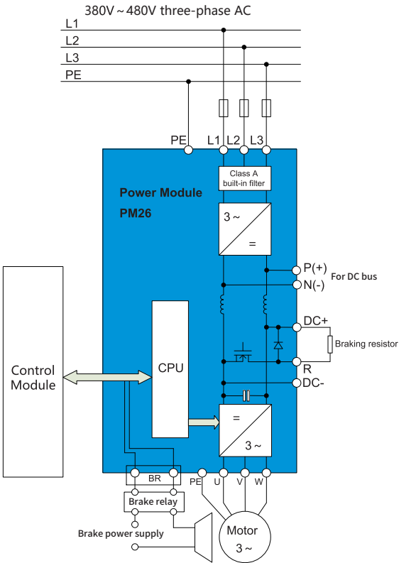
17.3 功率模块电气连接
